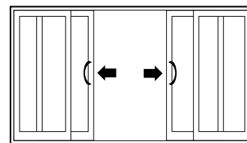
OXXO - Panneau central mobile vers la droite et vers la gauche
